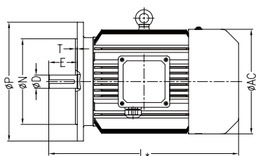
B5安装结构形式
