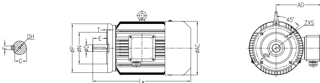
B14B 安装结构形式
