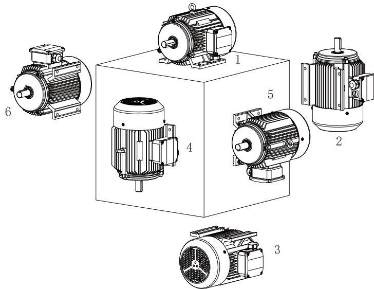
马达接线盒和进线孔 位置(视角: 马达尾部)
