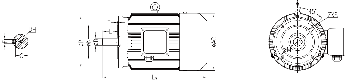
B14B 安装结构形式
