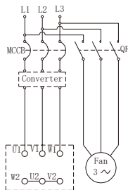
基础接线示意图
