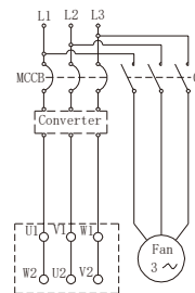
2) 配强冷风机马达 2) Forced-fan cooling motor
