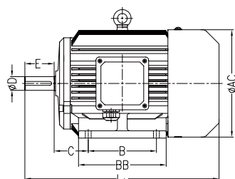
B3 安装结构形式
